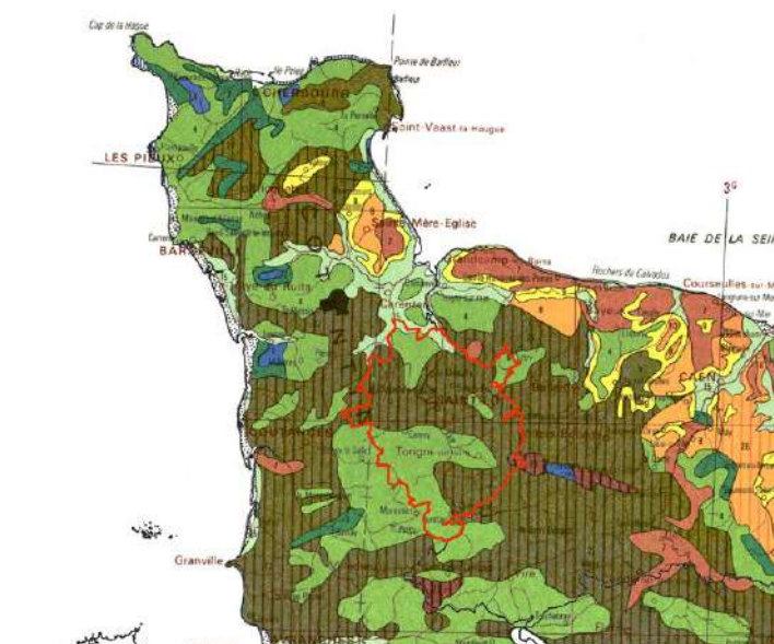
Carte géologique, les formations sédimentaires. Source : BRGM
