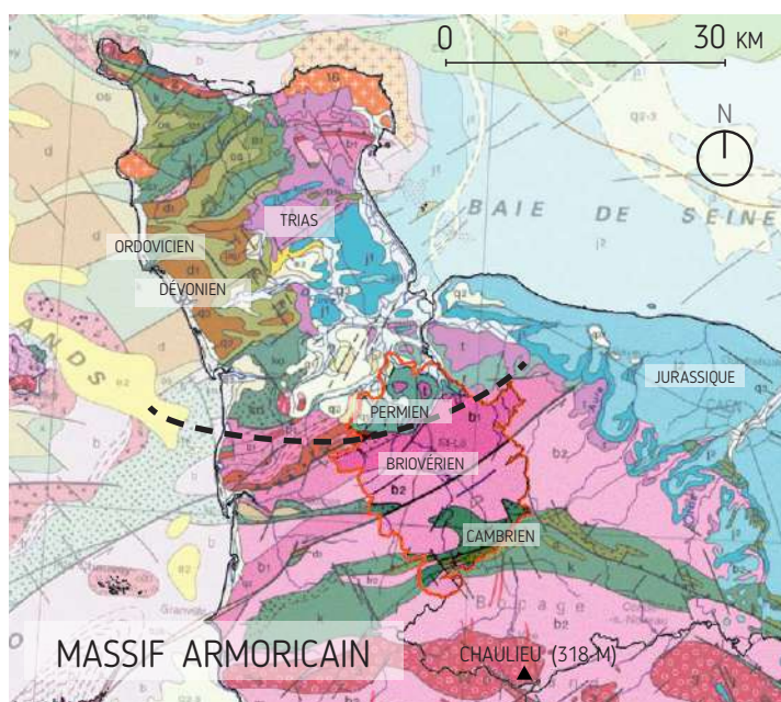
Carte géologique, les formations sédimentaires. Source : BRGM
